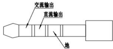
图 4-1-5 立体声插头引脚
