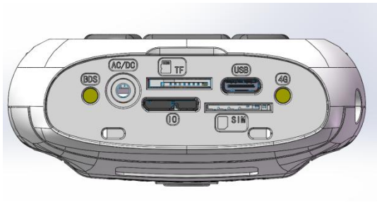
图 4-1-4 底部接口
