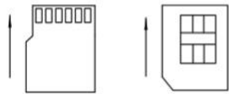
图 4-1-6 TF 卡与 SIM 卡的插入方式
