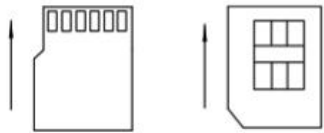
图 4-6 TF 卡与 SIM 卡的插入方式
