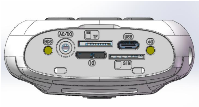
图 4-1-4 底部接口
